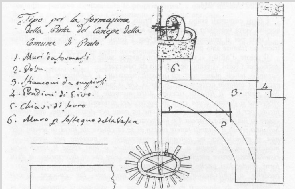
Disegno della Pista da canapa – 1807 (A.C.P.)
