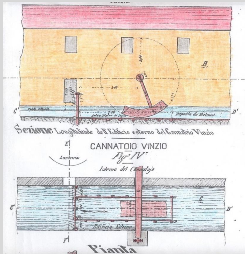
Ruota del filatoio – disegno di Paolo Valle – 1871 (A.S.N., disegni, Tribunale, TR V vol. 110/27.7, Mora 1871)
