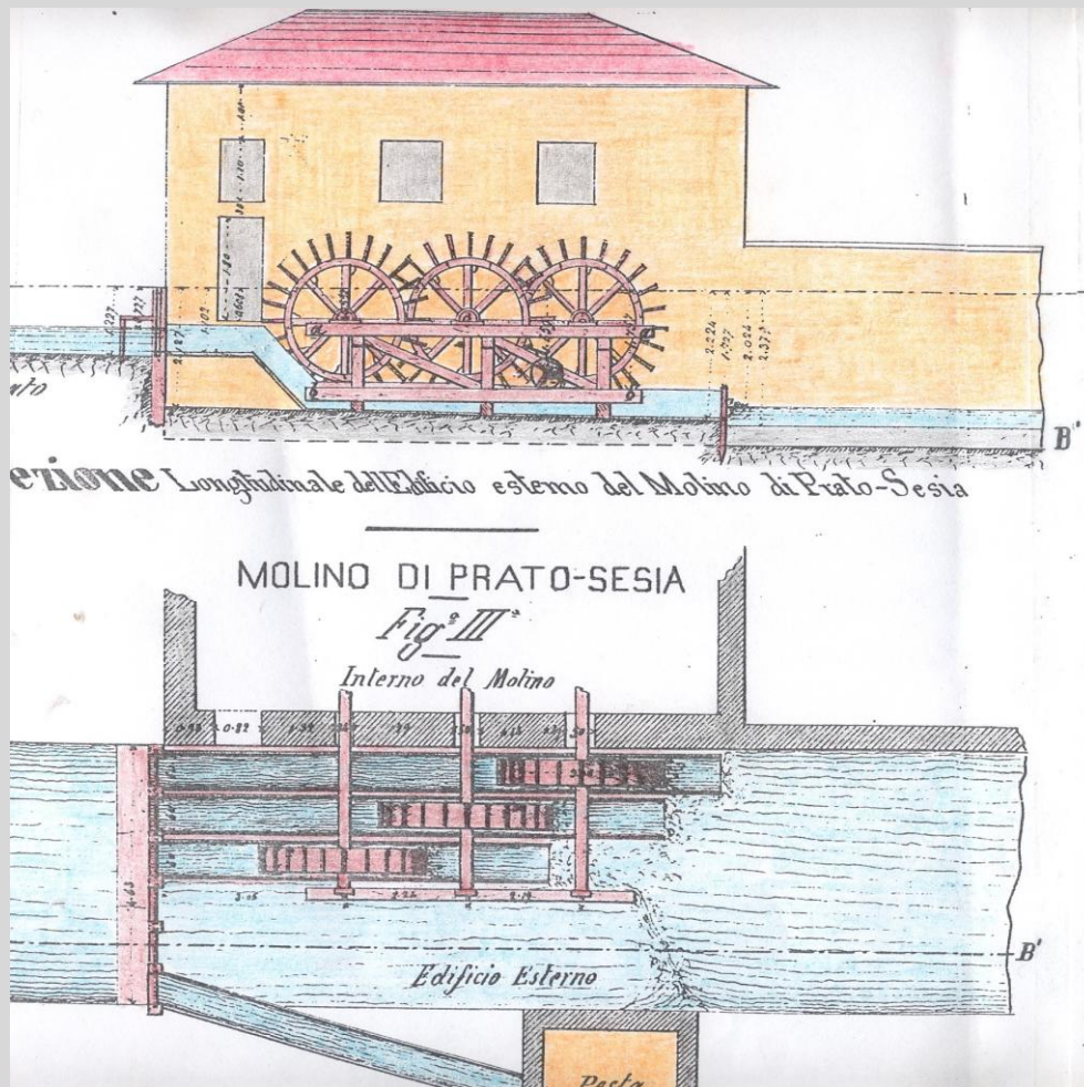
Disegno del Mulino Nuovo – Paolo Valle – 1871 (A.S.N., disegni, Tribunale, TR V vol. 110/27.7, Mora 1871)
