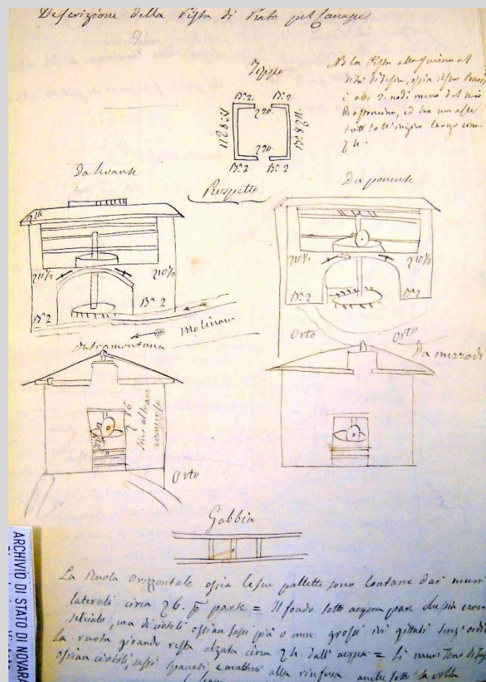
Disegno della Pista da canapa – 1821 (A.S.N., Archivio Bollati)
